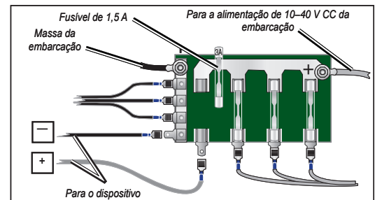
Exemplo de bloco de fusíveis
